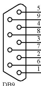
DB9
